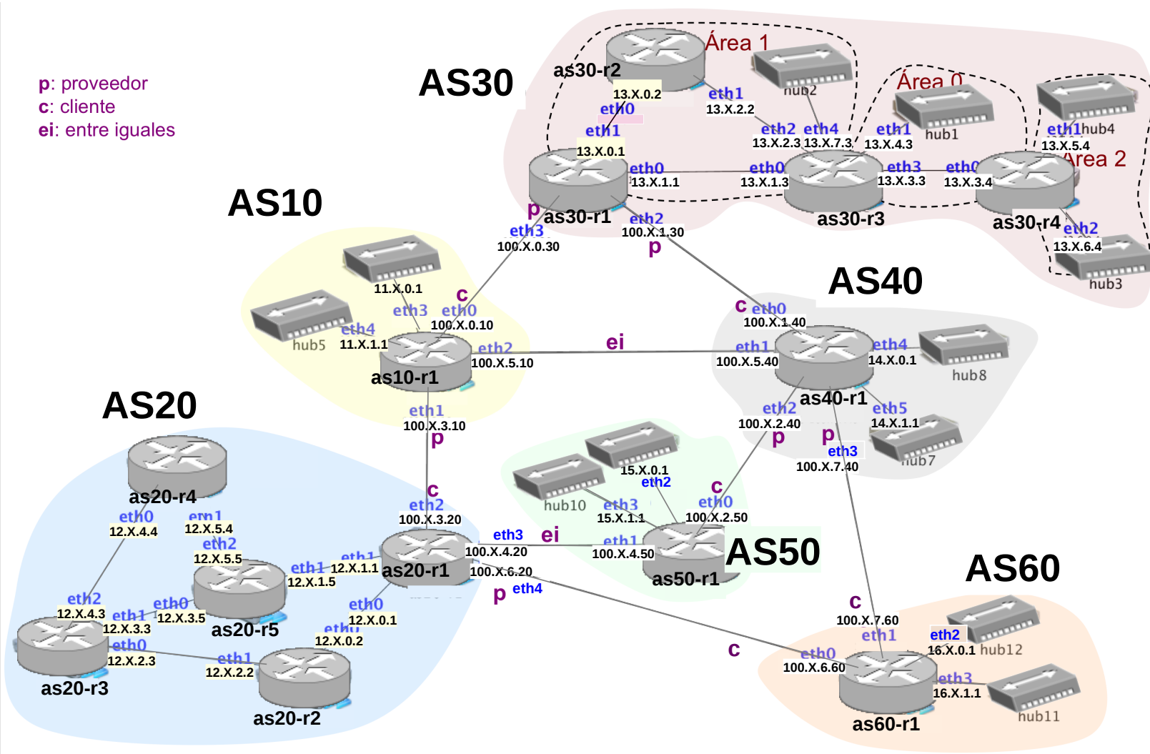
Figura 2: Escenario para listas de exportación y local pref en BGP
